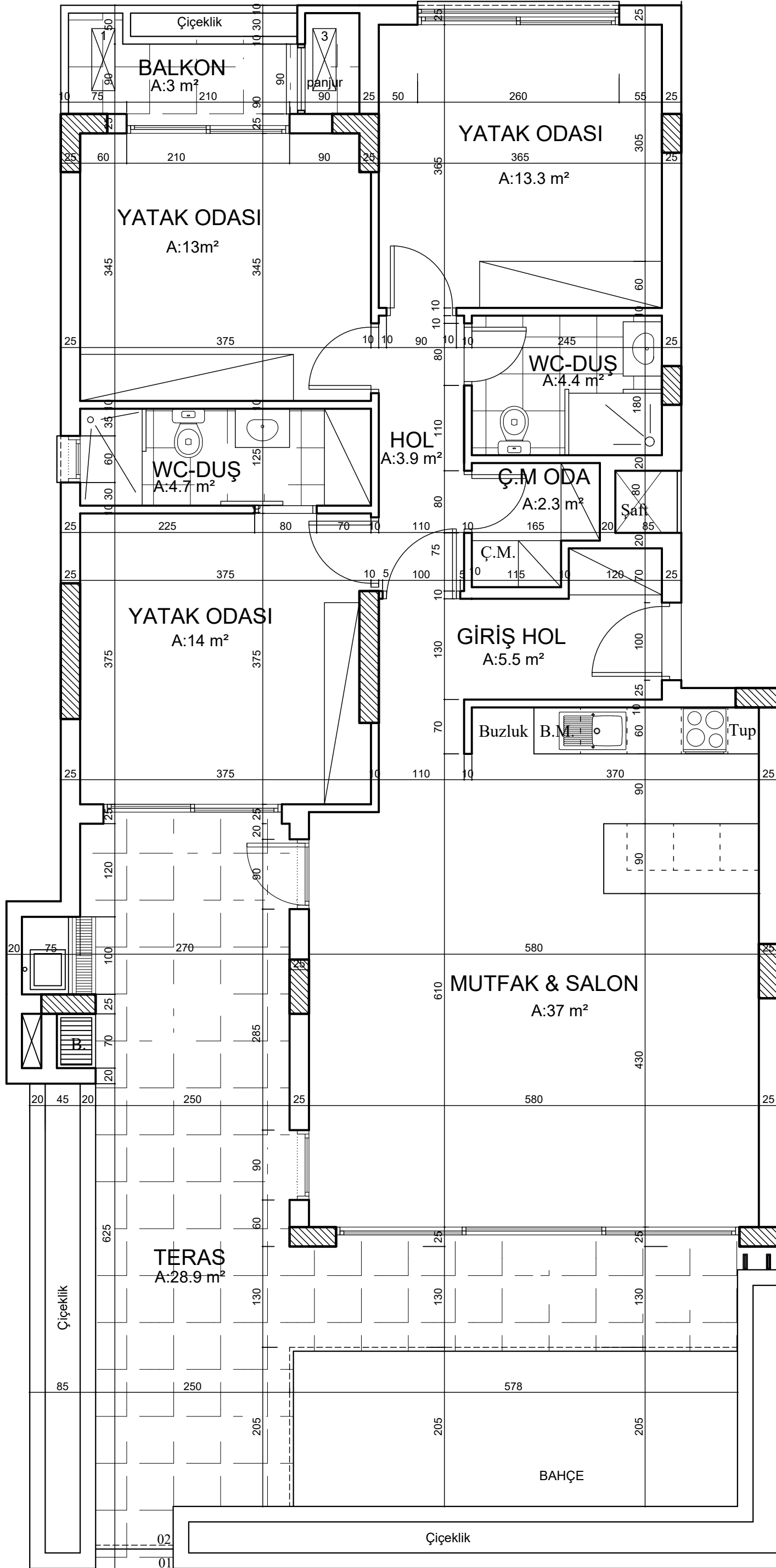
ZEMİN KAT 3+1
